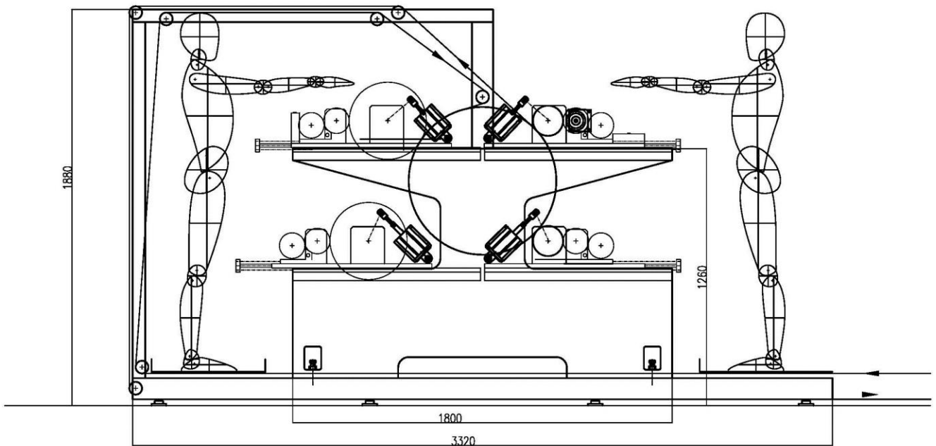
Рис.1 Схема печатного модуля
